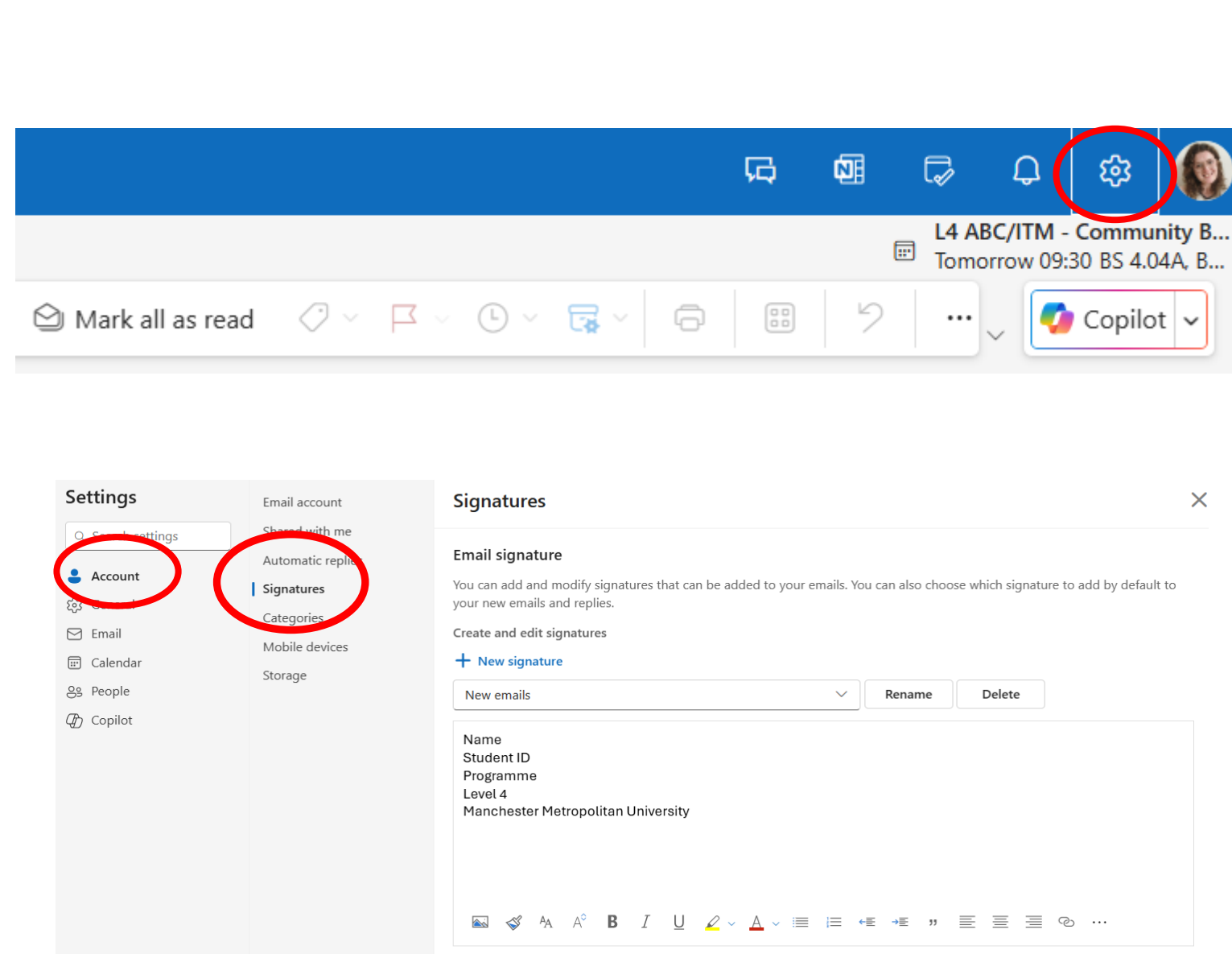
Web browser
